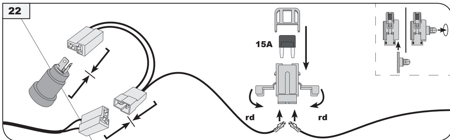
E-Satz → 12V Steckdosenleitungsstrang e-kit → 12V car power outlet
