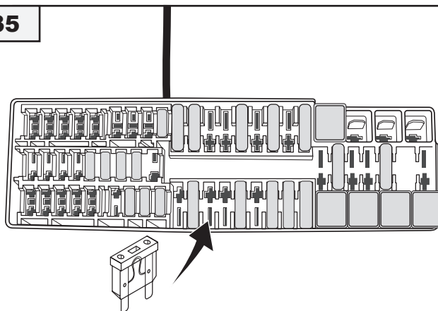
Sicherung 15A ➔ Kammer F8 fuse 15A ➔ fuseslot F8
