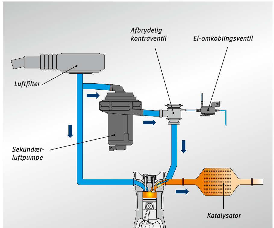
Sekundærluftsystem, skematisk
