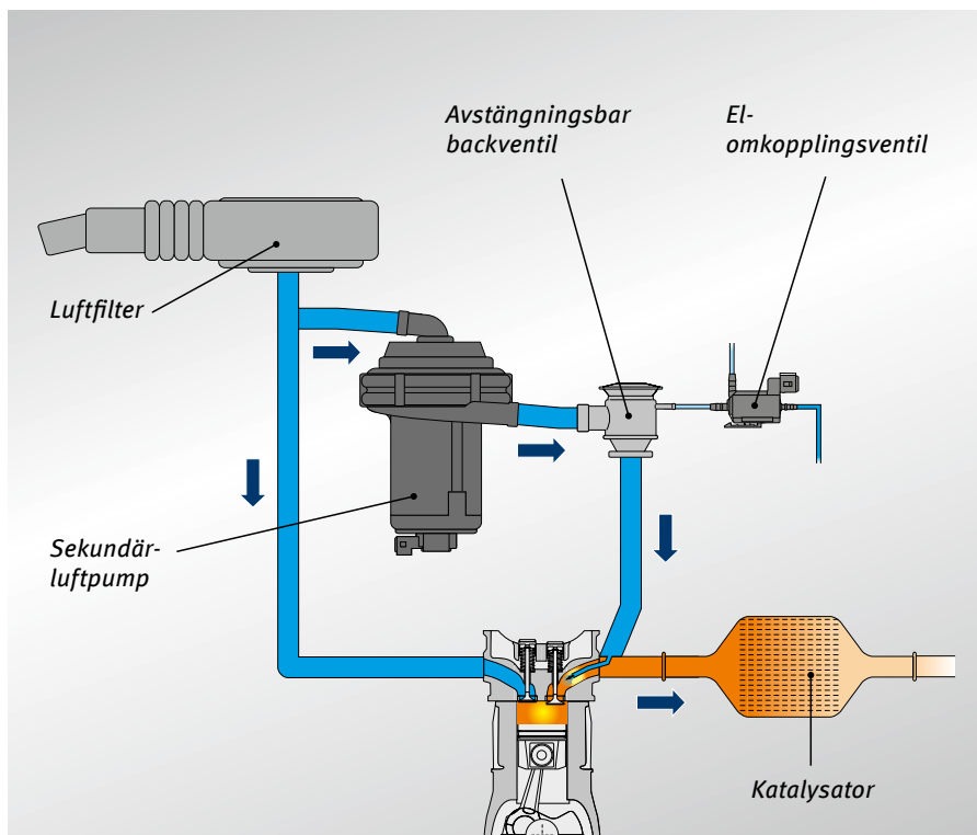
Sekundärluftsystem, schematiskt
