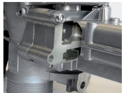
Κλαπέτο παράκαμψης στο ψυγείο EGR (τομή)
