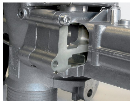
Байпасная заслонка в радиаторе системы EGR (в разрезе)
