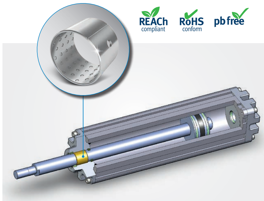
Anwendung Pneumatikzylinder, Lagerung mit Permaglide® P200 Gleitlager
