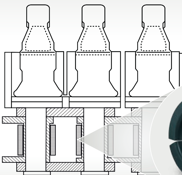
Supporto delle pinze con boccole langiate a strisciamento PERMAGLIDE® P10
