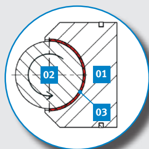
Anwendung Radialkolbenprinzip
