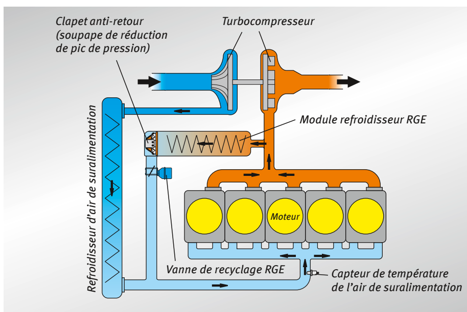
Schéma du recyclage des gaz d'échappement refroidis
