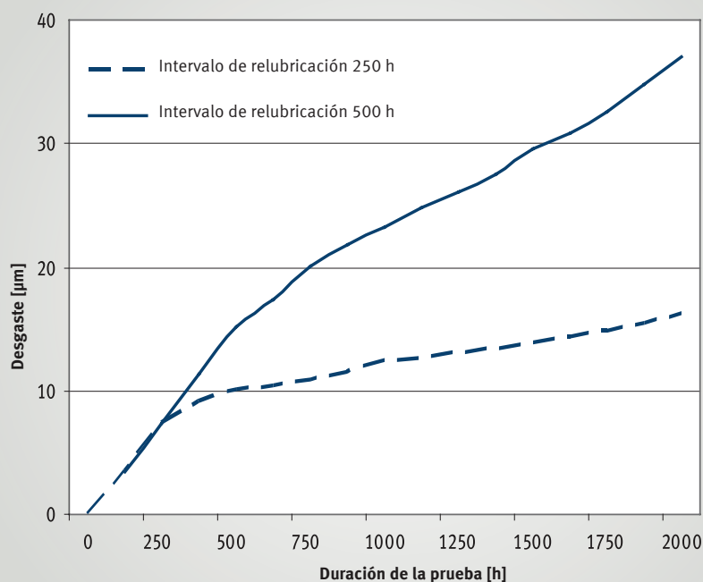
Curva de desgaste de cojinetes de fricción P2 (esquemática)
