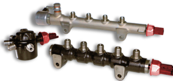
Capteurs de pression du carburant sur le rail (en rouge)
