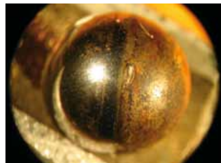
Rys. 7: Kulka zamykająca
