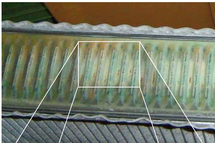
Rys. 1: Rozcięta chłodnica wodna
