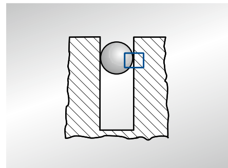
Rys. 4: Zatyczka kulkowa
