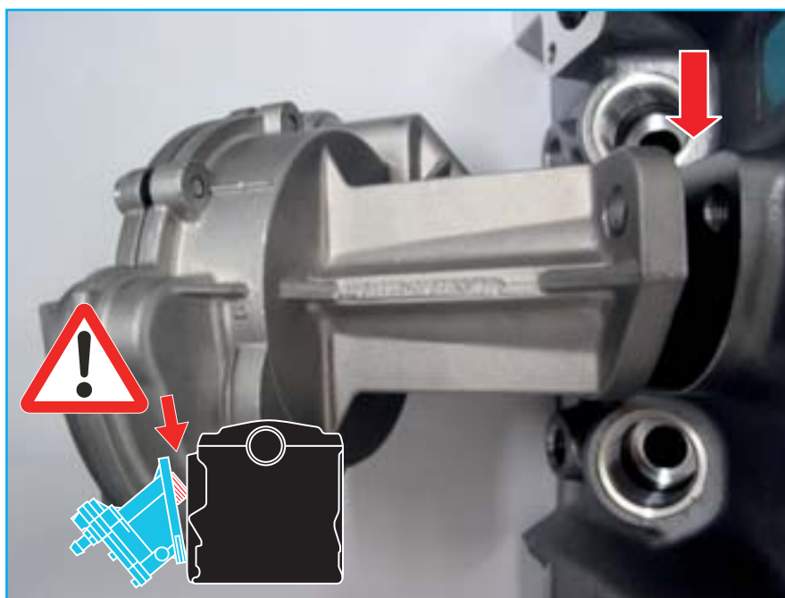
Fig. 5 V případě chybně zvoleného typu čerpadla nebude montáž možná
